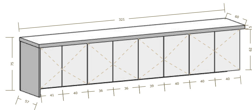
DETALHE 03 1:25
