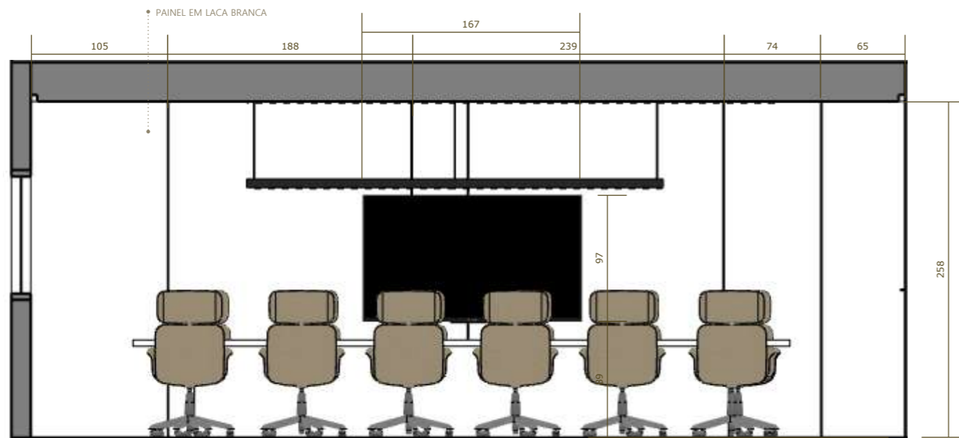
ELEVAÇÃO C 1:40
