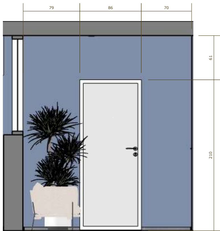
ELEVAÇÃO A 1:30
