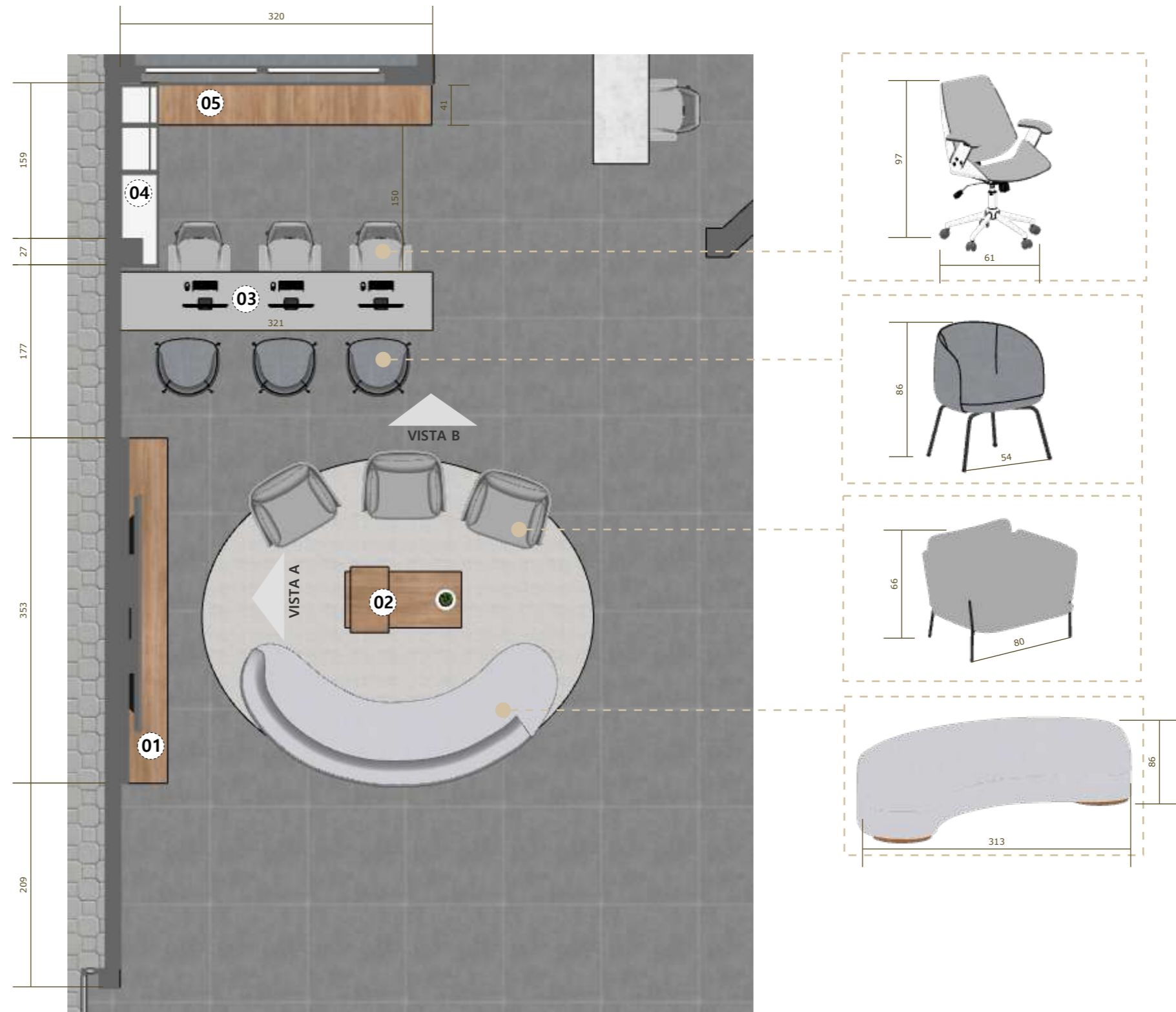
PLANTA HUMANIZADA 1:50
