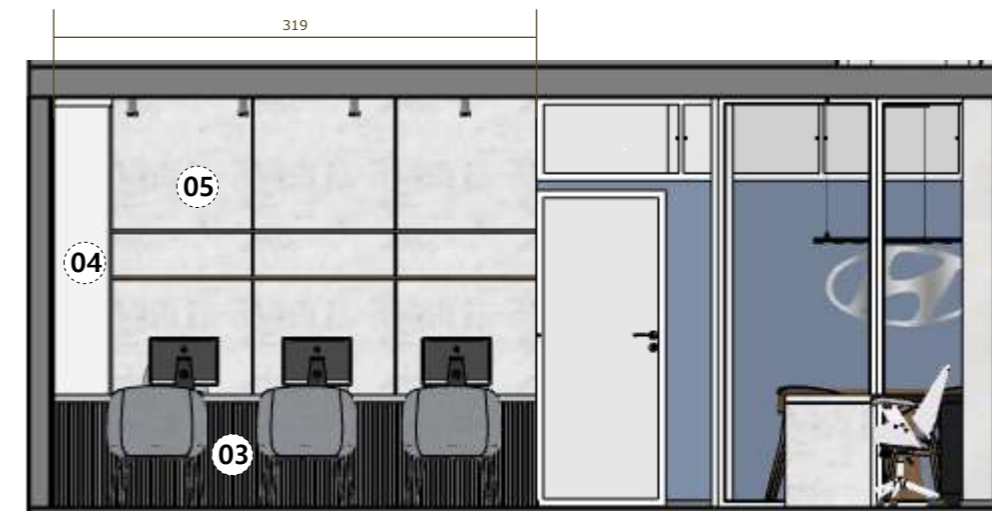
ELEVAÇÃO B 1:50
