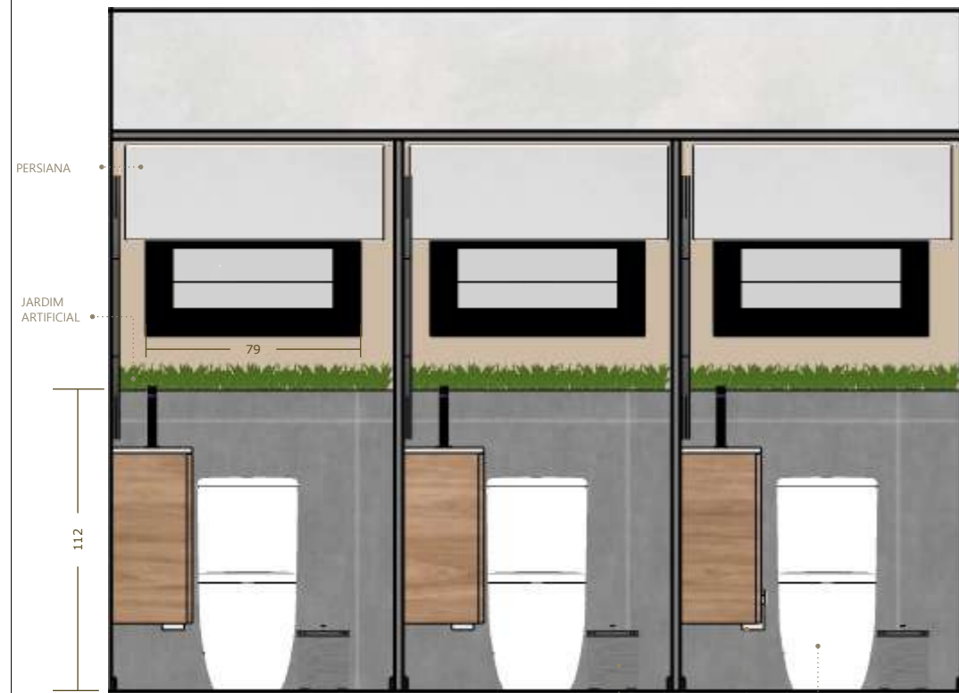
ELEVAÇÃO C 1:25
