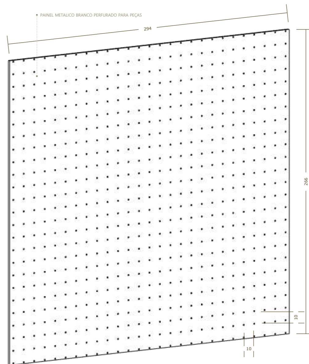
DETALHE 02 1:20
