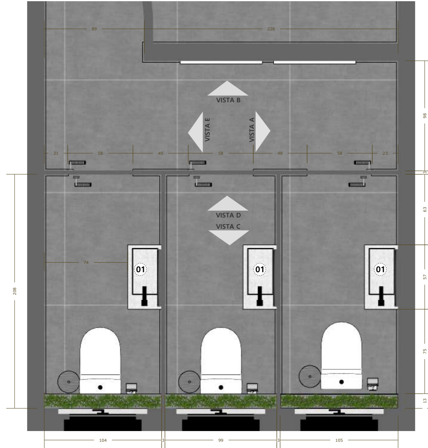
PLANTA HUMANIZADA 1:20
