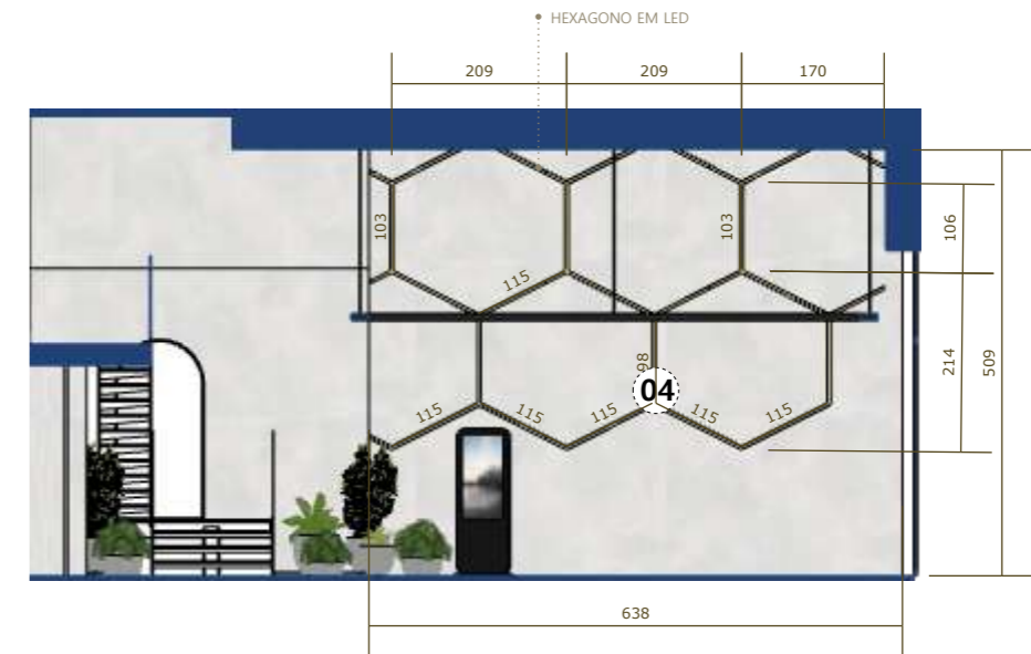
ELEVAÇÃO B 1:100
