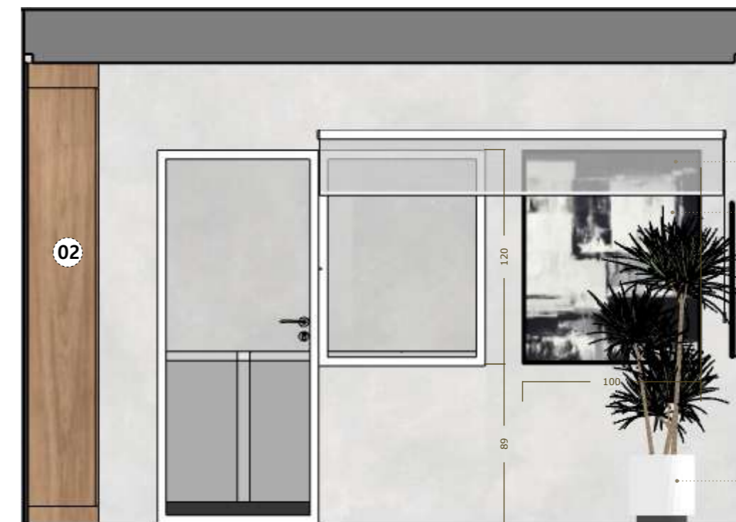
ELEVAÇÃO B 1:30
