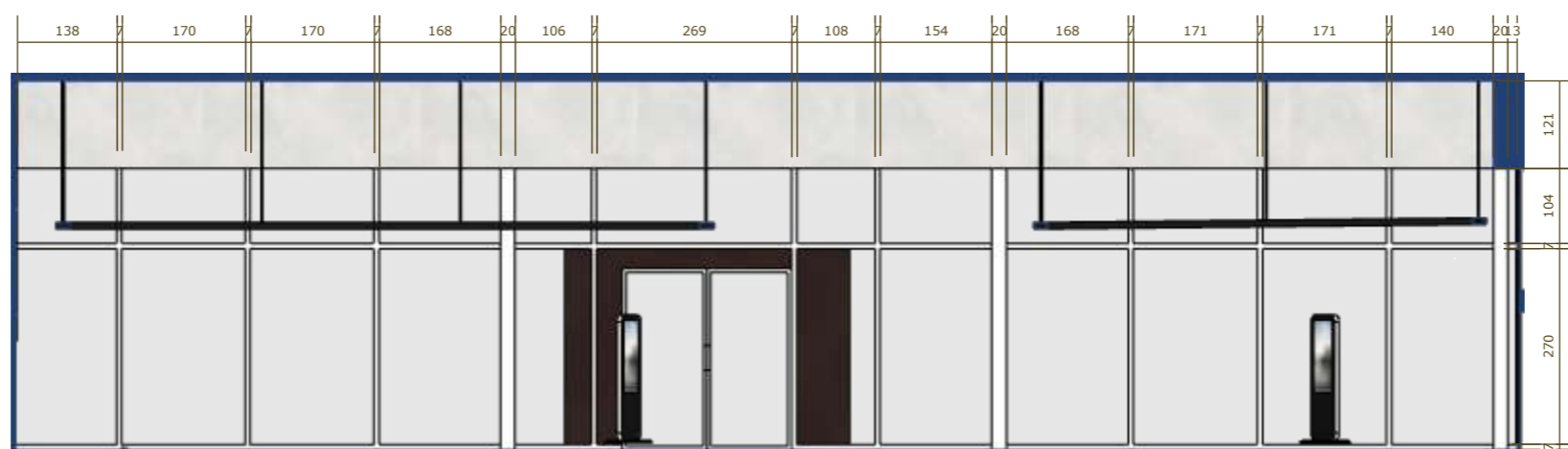
ELEVAÇÃO E 1:100
