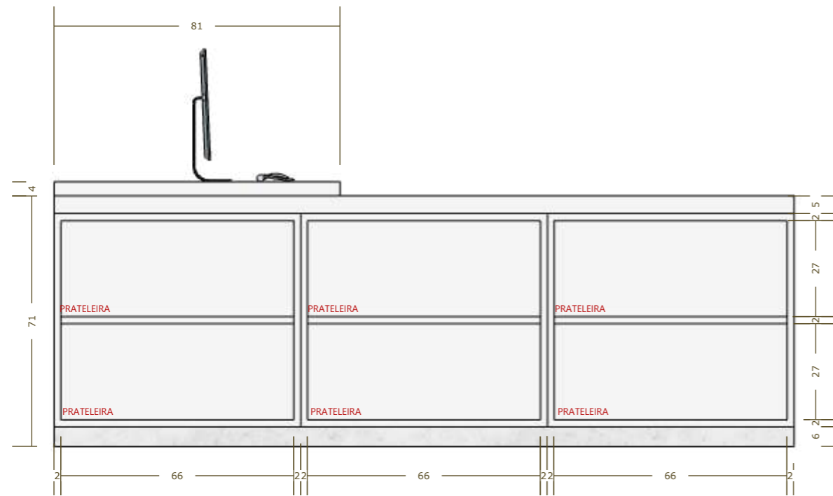
DETALHE 01 1:15
