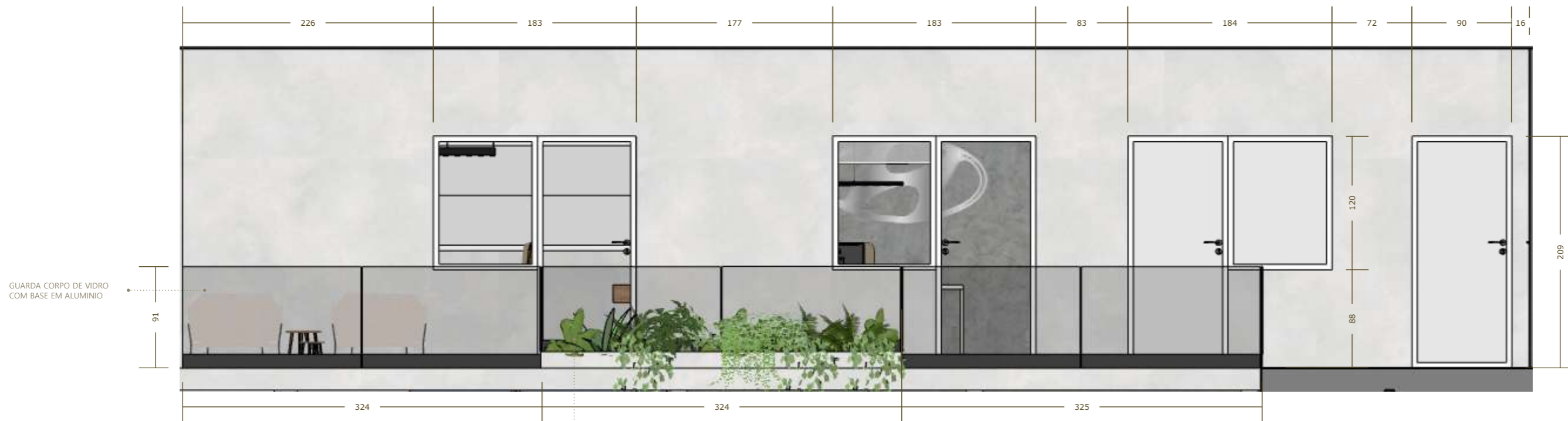
ELEVAÇÃO A 1:40
