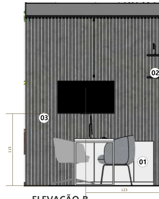
ELEVAÇÃO B 1:30
