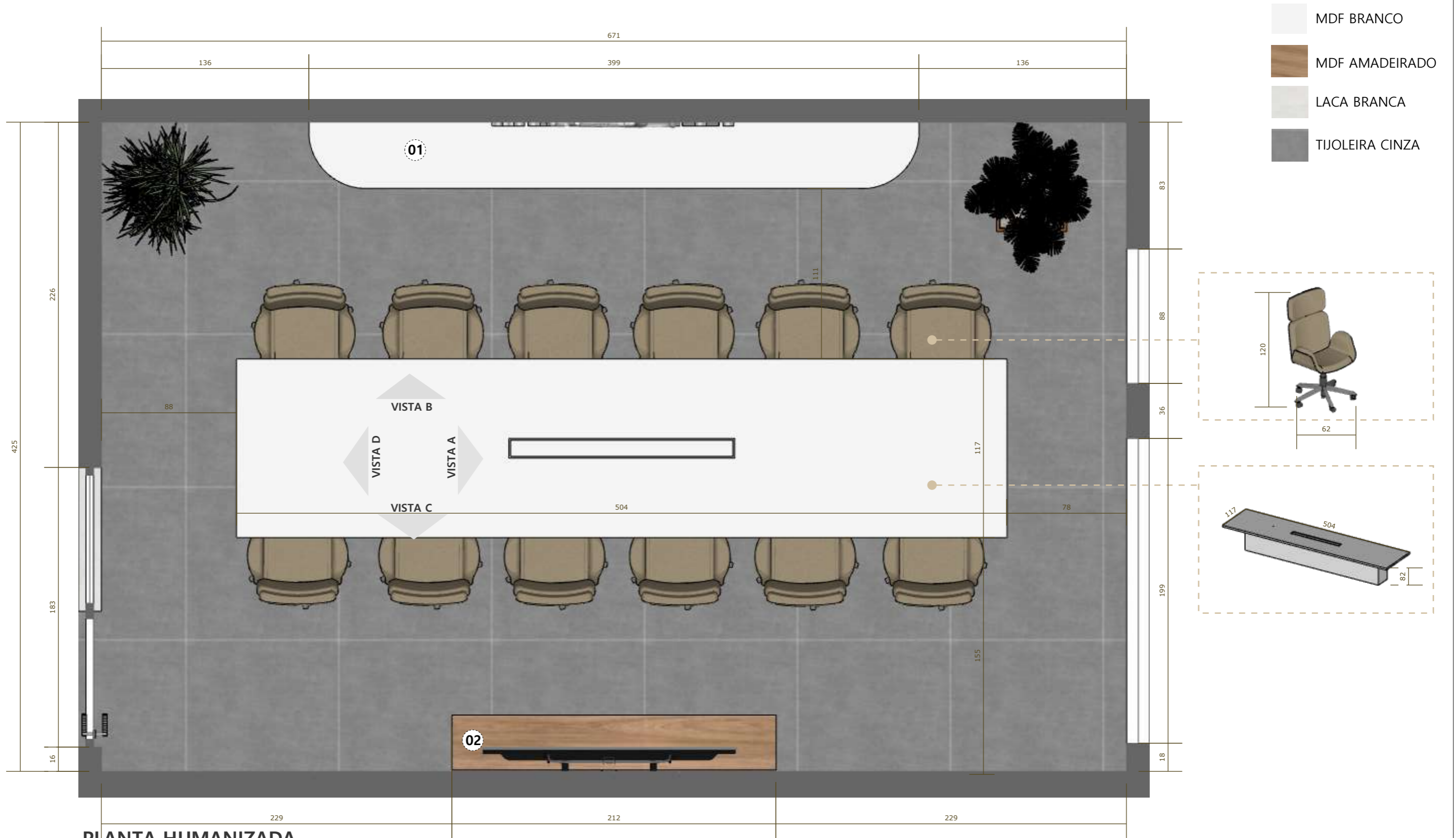
PLANTA HUMANIZADA 1:25
