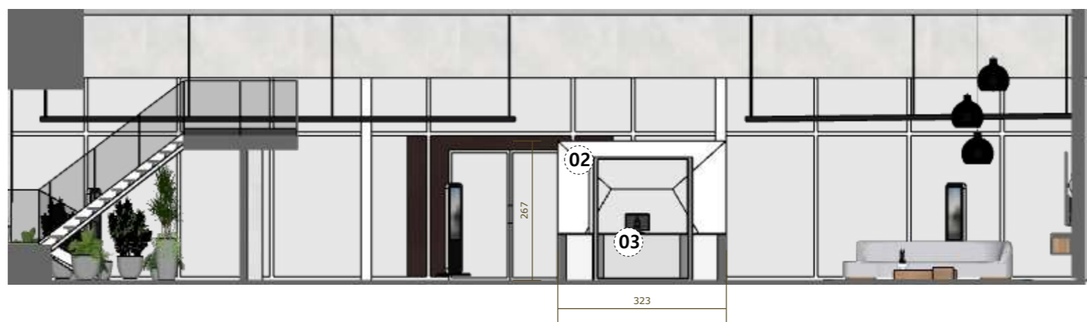
ELEVAÇÃO F 1:100
