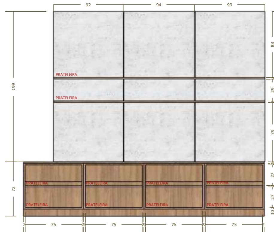
DETALHE 05 1:30
