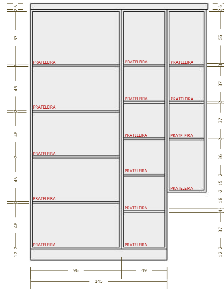
DETALHE 04 1:25
