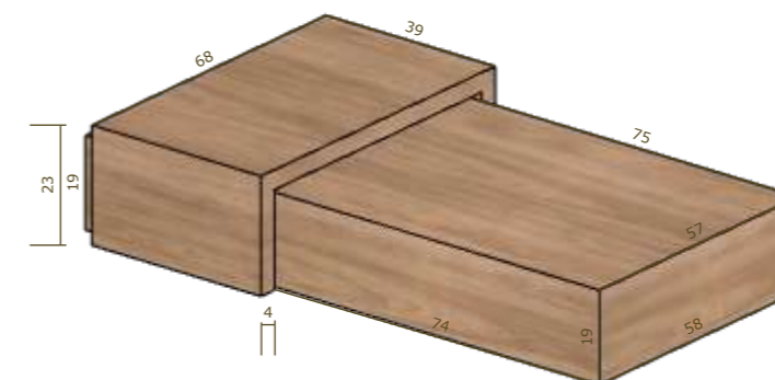
DETALHE 02 1:15
