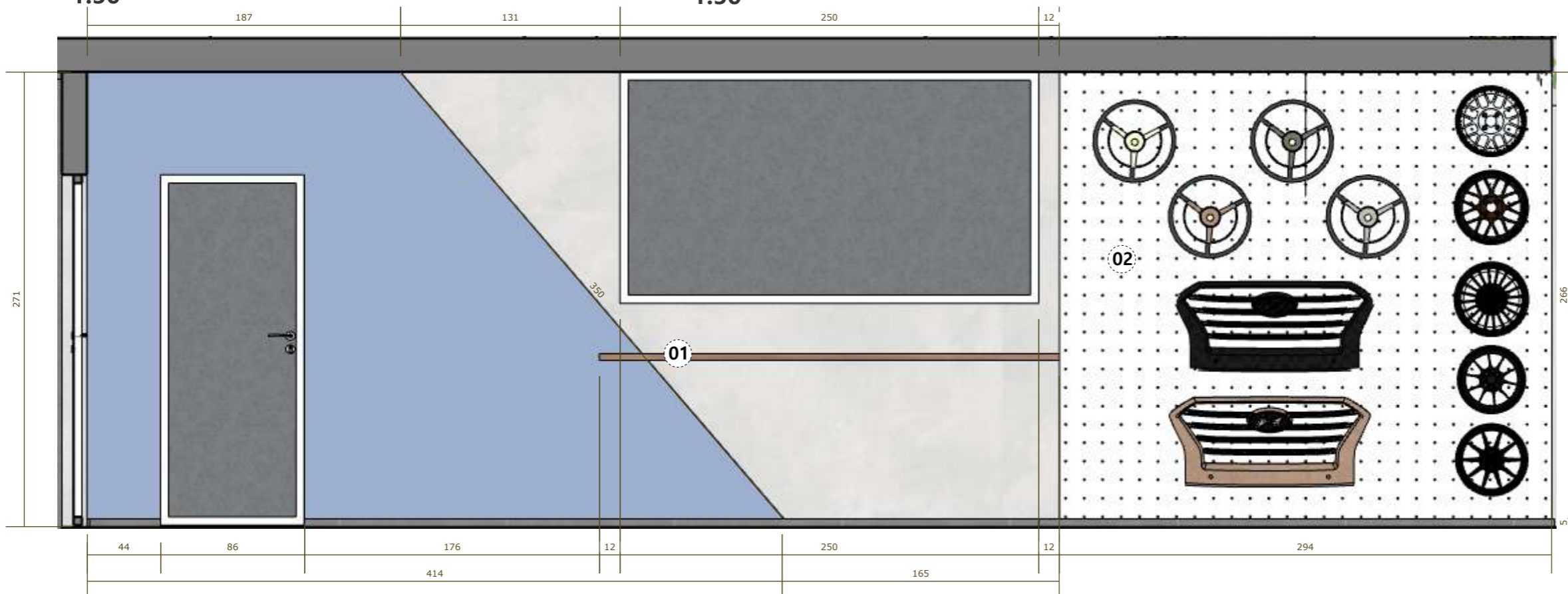
ELEVAÇÃO A 1:30
