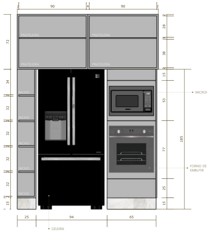
DETALHE 04 1:25
