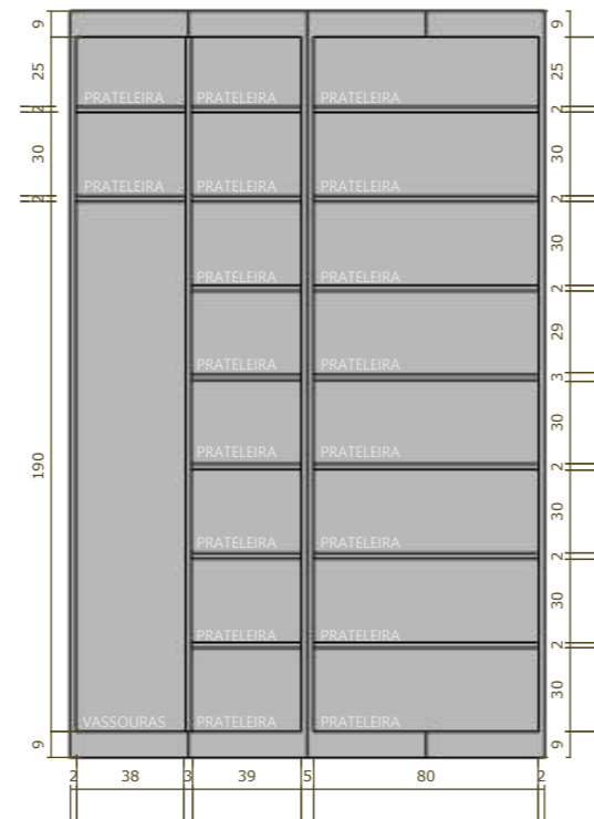
DETALHE 08 1:30
