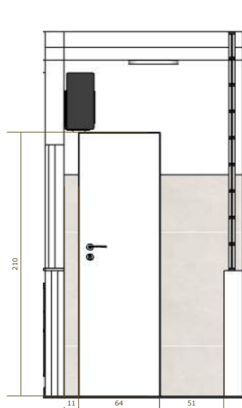
ELEVAÇÃO L 1:30
