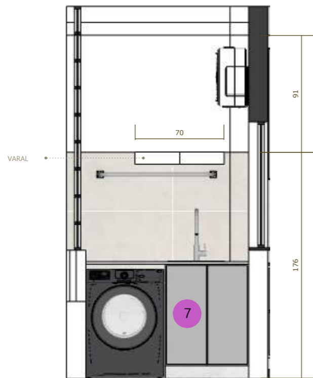
ELEVAÇÃO N 1:30
