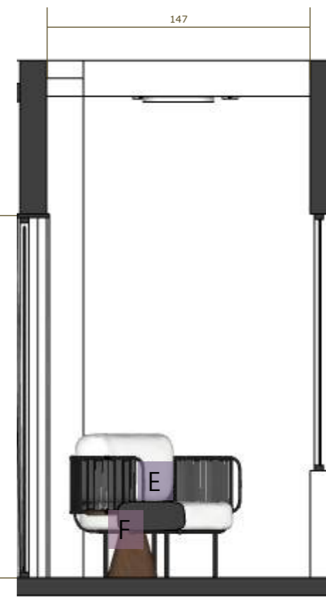
ELEVAÇÃO G 1:30
