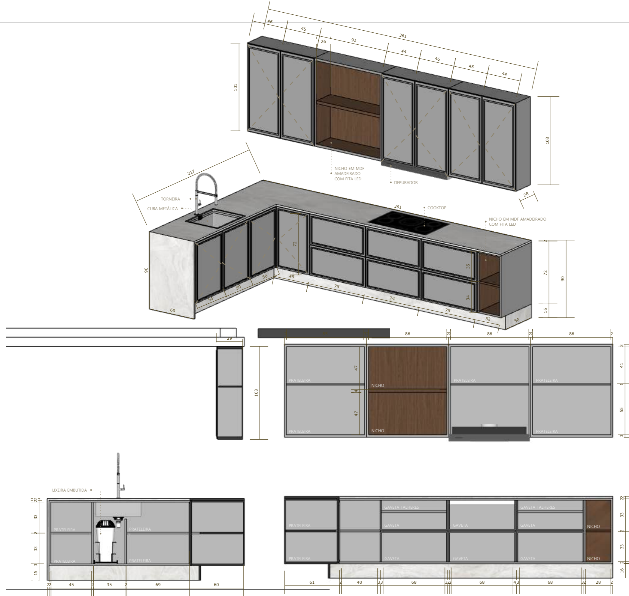
DETALHE 06 1:25
