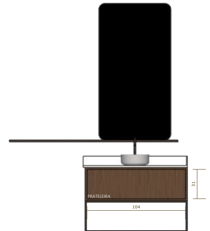
DETALHE 10 1:25
