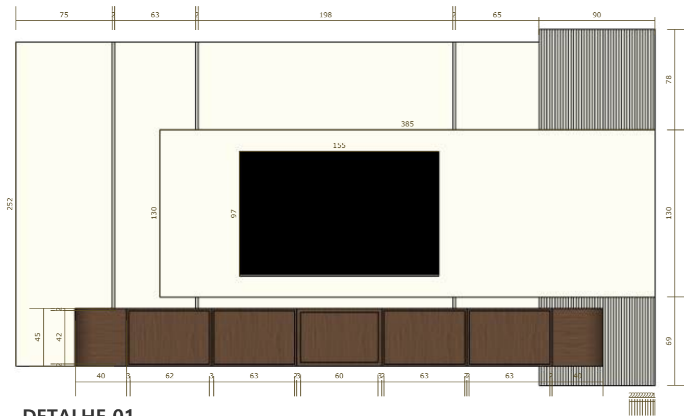
DETALHE 01 1:30
