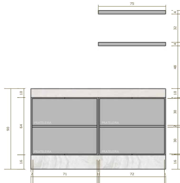
DETALHE 09 1:20
