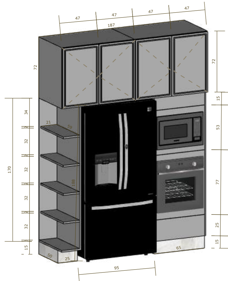
DETALHE 03 1:25
